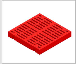
PS-M-1644 Aleta P/ Módulo Trommel 12" x 12" abert. 10 x 60 mm
