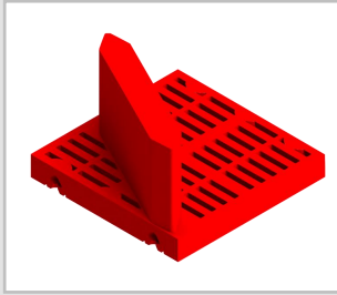
PS-M-1642-1 Módulo para Trommel 12" x 12" abert. 10 x 60 mm c/Aleta
