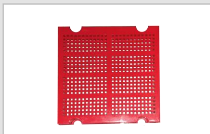
PS-MM-876 Módulo de Poliuretano p/ Criba, 12" x 12" con abert. de \frac{1}{4} " x \frac{1}{4} "
